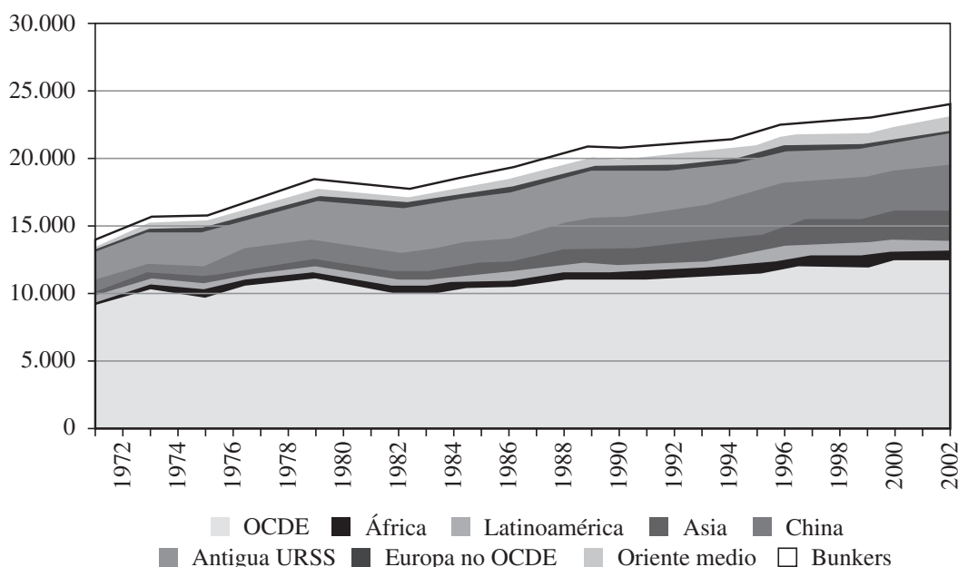
Gráfico 3. Emisiones de CO 2 en el mundo por regiones (Mt CO 2 ), 1971-2002
