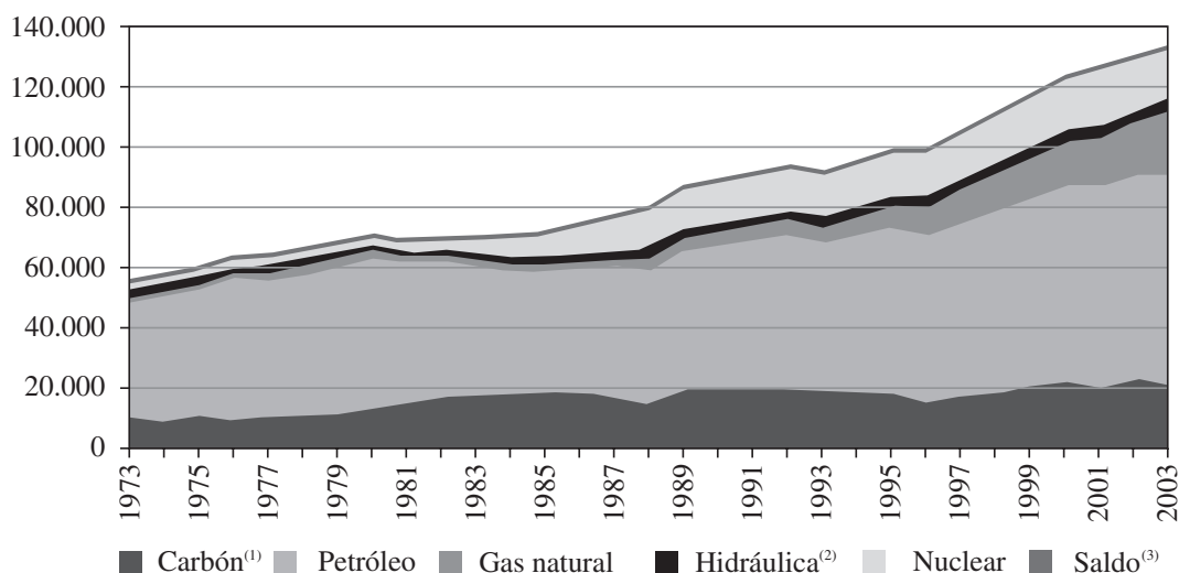
Gráfico 4. Consumo de energía primaria en España, por fuentes de energía (ktep)
